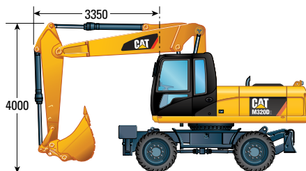
Положение для движения по дорогам, с рукоятью 2500 мм
