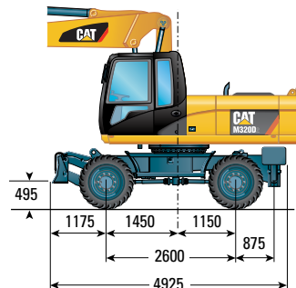
Ходовая часть, оснащенная 1 комплектом опор и отвалом
