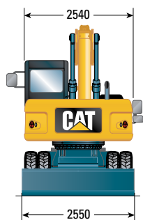
Положение для движения по дорогам, с рукоятью 2500 мм
